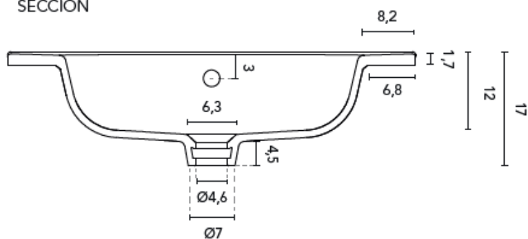
SECCIÓN
