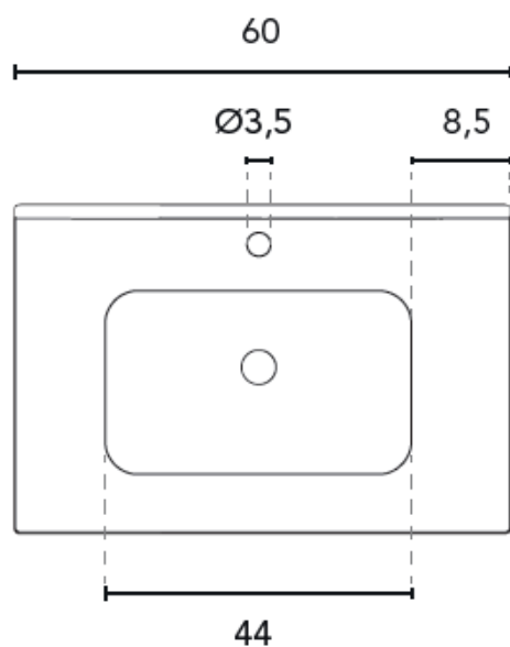
PLANO MUEBLE LOTO 60 CM
